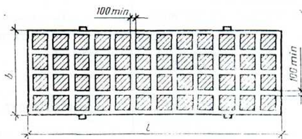
Расположение нагрузки на плите в плане
