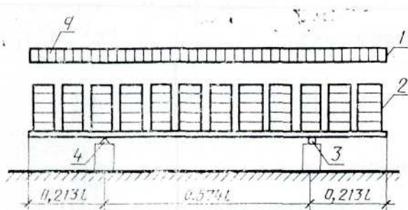
Схема опирания плиты
