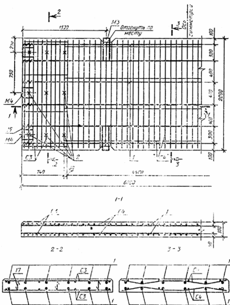
1 — напрягаемая арматура; 2 — крепление сеток С3
