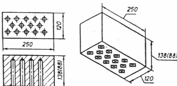
Рисунок А1 — Камень (кирпич) 14-пустотный (диаметр отверстий 30—32 мм, пустотность 28—31%)
