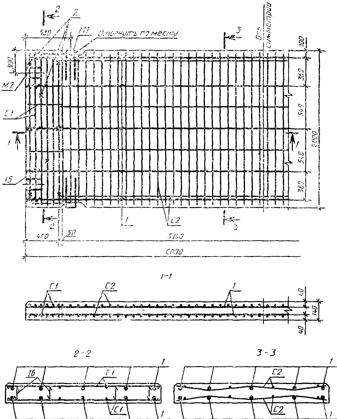
1 — напрягаемая арматура; 2 — крепление сеток C1
